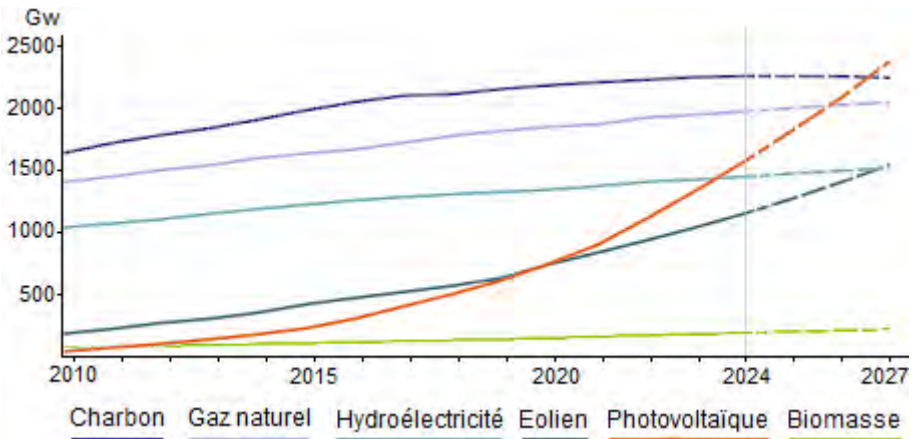
Figure 2 : Évolution des capacités de production d'électricité d'ici 2027 selon le scénario central de l'AIE
