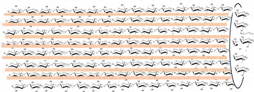
Figure 27 : État pseudo-cristallin engendré par les liaisons hydrogène inter-caténaires (représentées en couleur saumon)
