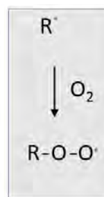
Figure 33 : radicaux peroxydes obtenus par oxydation de radicaux libres
