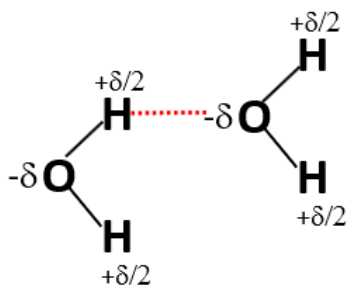
Figure 26 : Liaison hydrogène entre deux molécules d'eau \text{H}_2\text{O}
